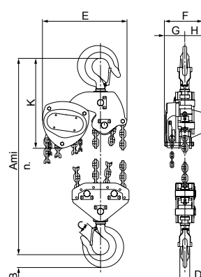
Modell VS///, 10000kg, 4-part
