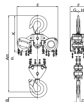
Modell VS///, 20000 kg, 8-part
