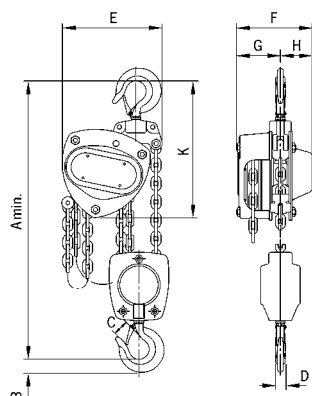
Modell VS///, 2000-5000kg, 2-part
