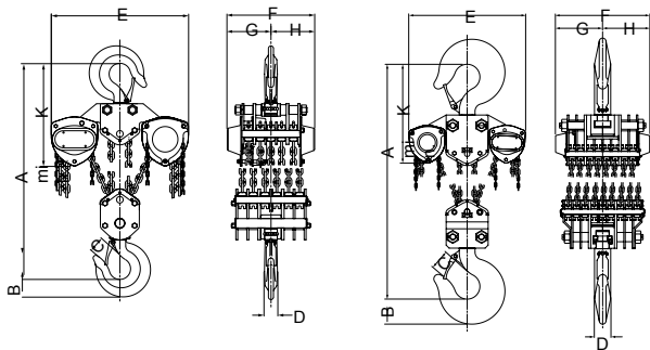
Modell VSIII, 50000kg, 18-part
