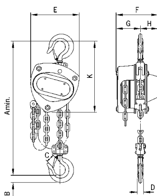
Modell VS///, 250-3000kg, 1-part
